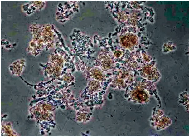
活性汚泥が分散し、原生動物が消滅している。
