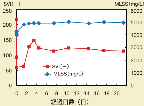
薬剤適用後の沈降圧密性推移
