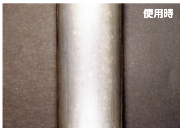
MC-2600 2000mg/L 添加。スケールの付着なし
