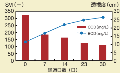
薬剤適用後の沈降圧密性及び透視度推移
