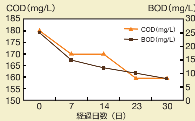
薬剤適用後の処理水質推移
