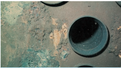
水管ボイラに発生した腐食
