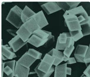
スケール生成時の結晶の粒子
