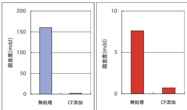
軟鋼 東京都2倍相当水
