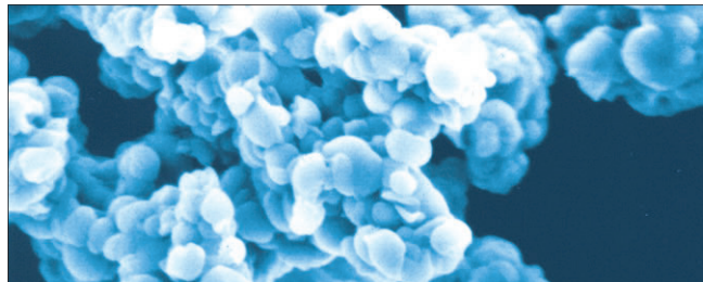
アクアスキレート D-205L 100mg/L 添加による結晶破壊の様子
