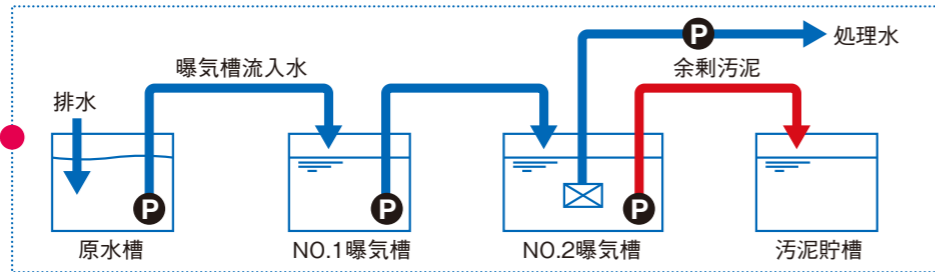
膜分離式活性汚泥処理設備 アクアスビオマスク
