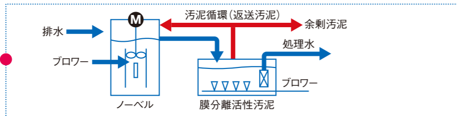
高効率好気性排水処理装置 アクアスノーベル
