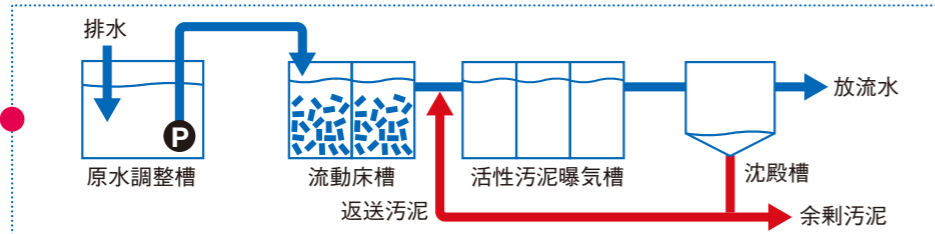
流動床式排水処理設備 バイオネスト
